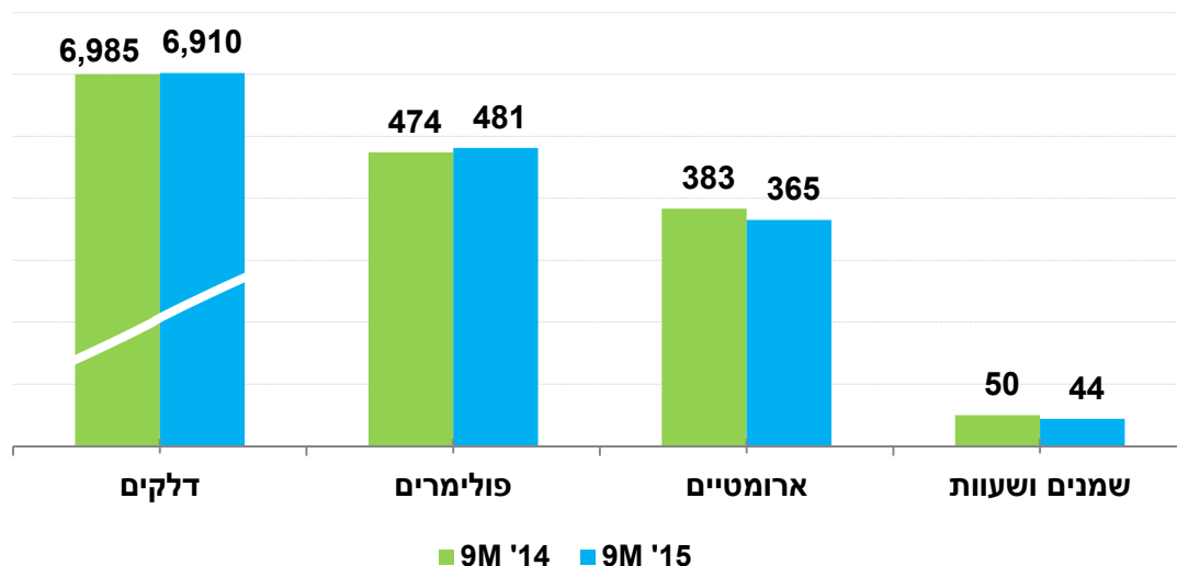
תשומה לזיקוק ותפוקת פטרוכימיה – אלפי טון
